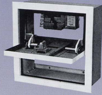
排煙口(N-961型)
